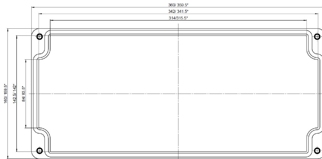
Deckel / Lid
